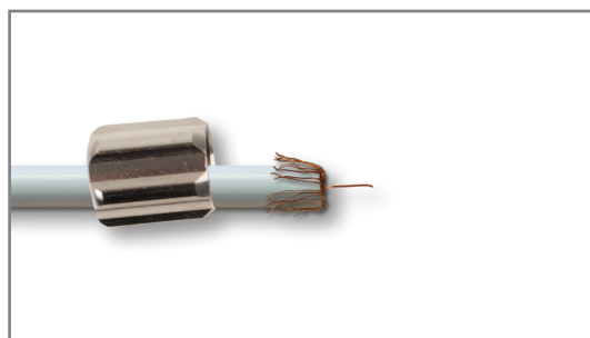
4) Plaats de connectorkap over de kabel. Slide the connector cap onto the cable.
