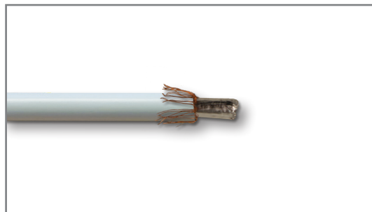
2) vouw de braiding terug over de mantel. De braiding mag niet met de vingers worden aangeraakt. Gebruik hiervoor het borsteltje van de CST 5 kabelstripper/mesje. Fold back the braiding. The braiding must not be touched with the fingers. To do this, use the brush of the CST 5 cable stripper/knife.
