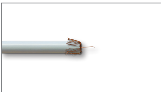
3) Verwijder het diëlektricum. Remove the dielectric.
